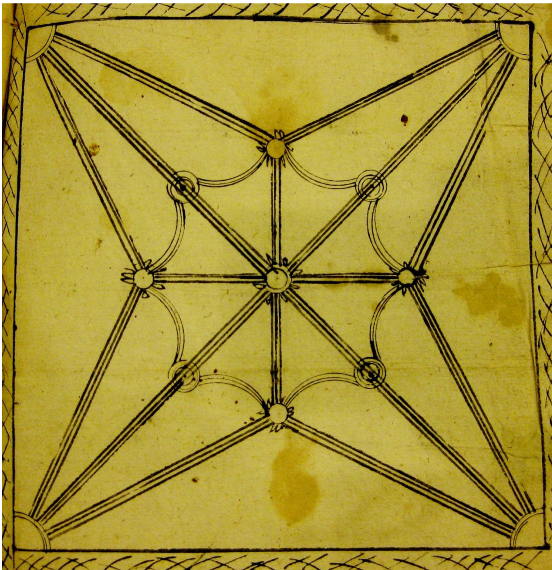
Fig. 3: Bóveda de la capilla de San Juan en la iglesia parroquial de la Asunción de Novales, según diseño del 10 de abril de 1638 de Felipe de Orna Rubalcaba.
