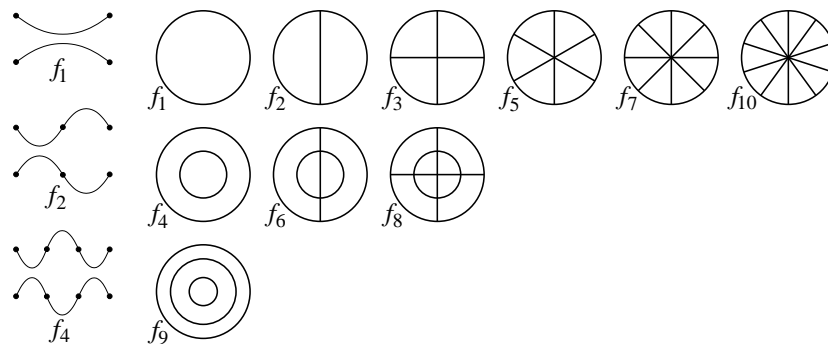
Figuro 2: Nodoj de la unuaj dek modoj de vibro de membrano. Maldekstre ni montras flanke membranon vibrantan laŭ modoj f_1, f_2 kaj f_4 .
