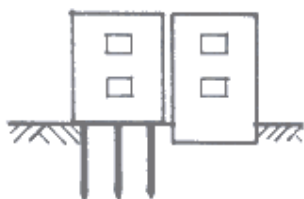
c. Sistemas de fundação diferentes.
