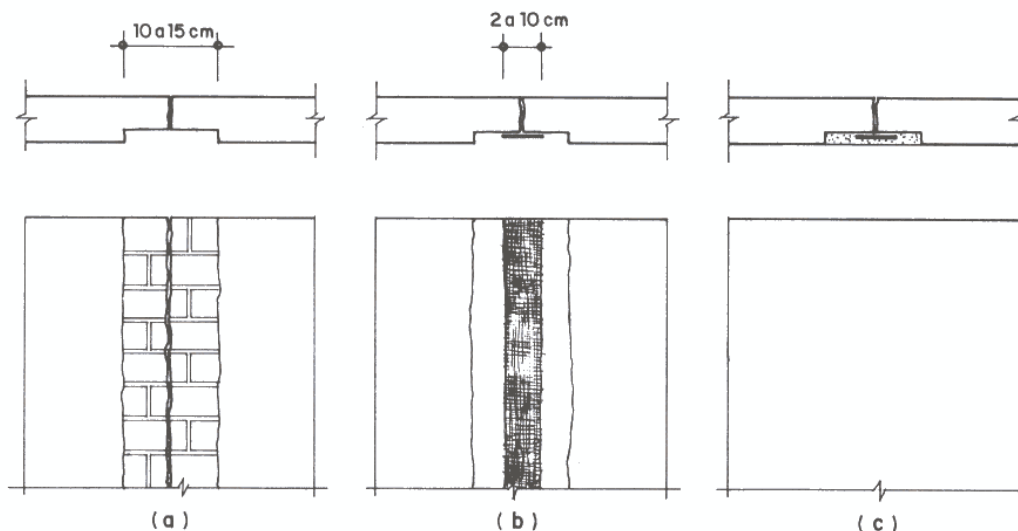
Figura 10. Recuperação de fissura em alvenaria por bandagem.
