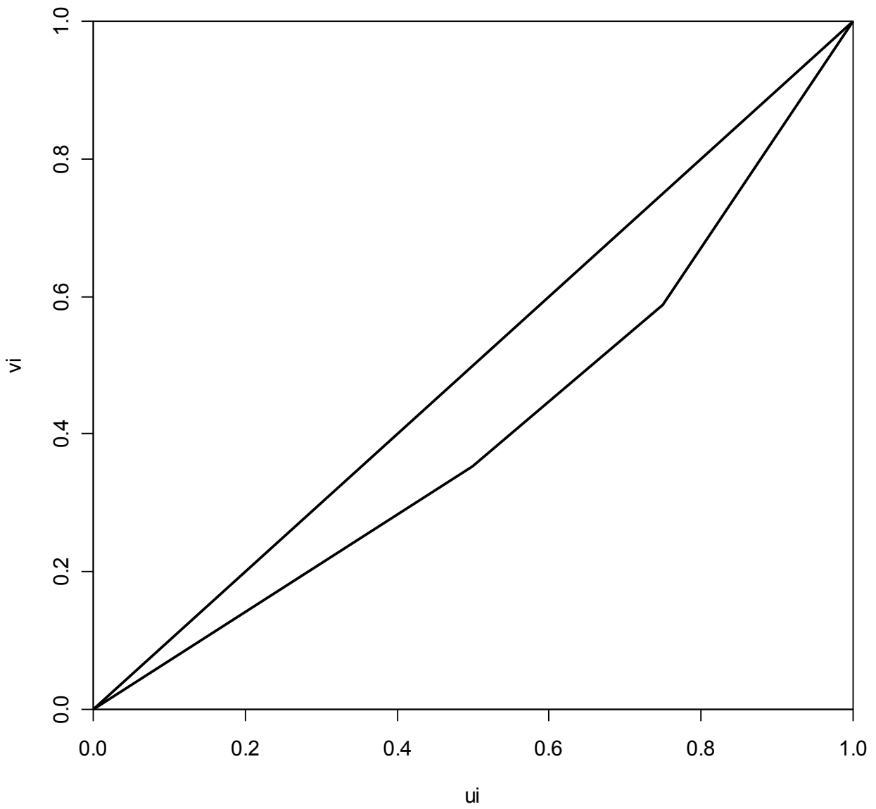
Lorenz-Kurve
