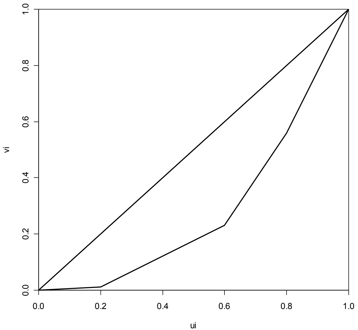
Lorenz-Kurve
