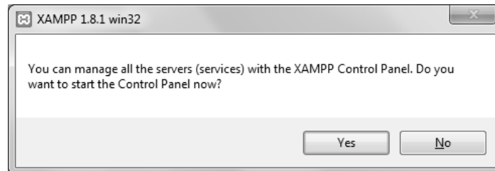
Gambar 1.17 XAMPP peringatan
