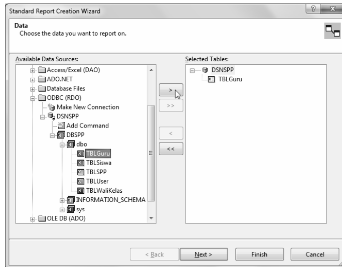
Gambar 3.19 Memilih tabel
