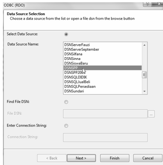
Gambar 3.17 Memilih DSN
