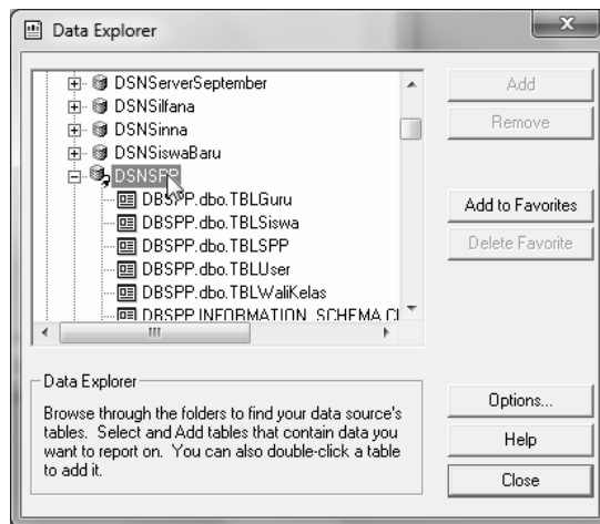
Gambar 3.5 Memilih DSN
