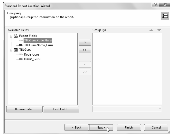
Gambar 3.21 Mengelompokkan data
