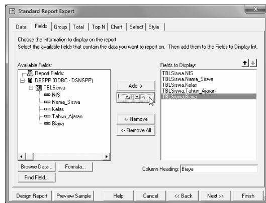
Gambar 3.8 Memilih field
