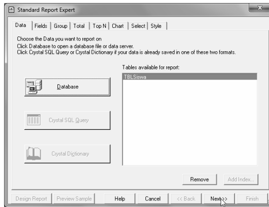
Gambar 3.7 Melanjutkan pilihan
