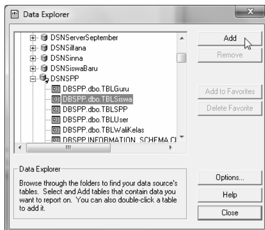
Gambar 3.6 Memilih tabel
