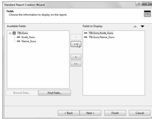
Gambar 3.20 Memilih field
