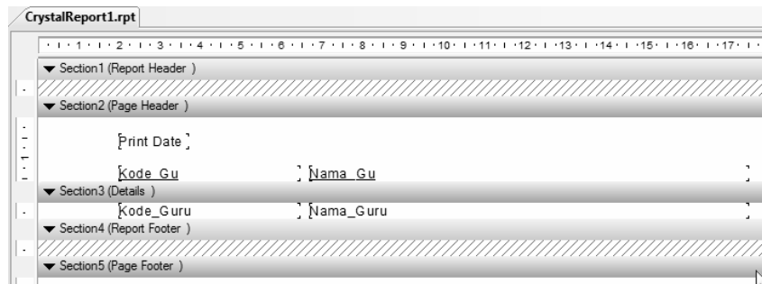
Gambar 3.23 Hasil laporan
